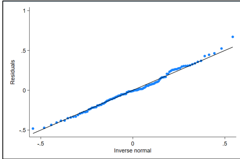
Görsel 1. Artıkların Normal Dağılım Uygunluğu
