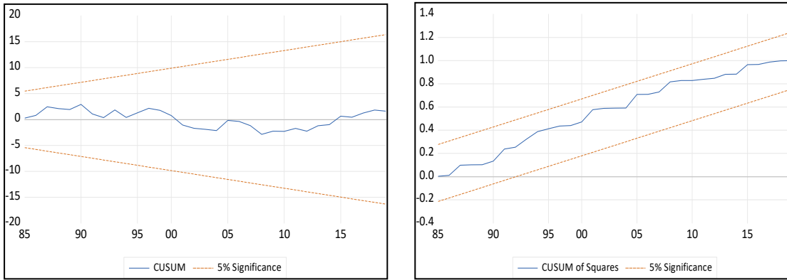
Grafik 1. CUSUM ve CUSUM 2 Test sonuçları
