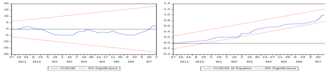
Görsel 3. ARDL(4,1): Kararlılık Testleri (OTOKAR - USD/TRY)
